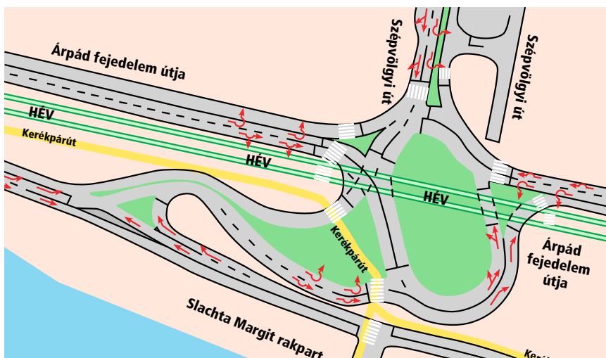
Az egyik javasolt változat a csomópont kialakítására
